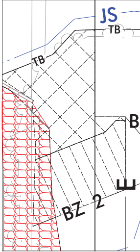
SITE I (14+39 -L- TO 15+04 -L- RT)
