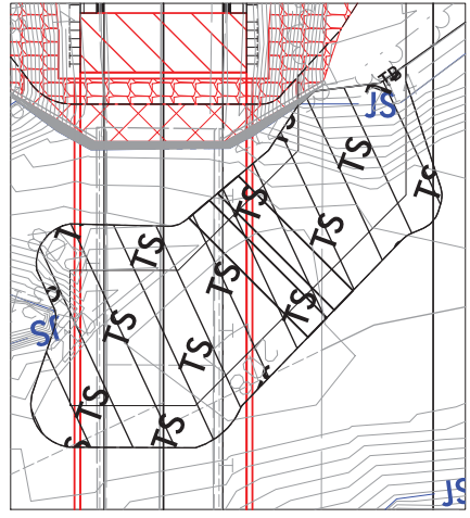
SITE I (15+10 TO 15+80 -L-)
