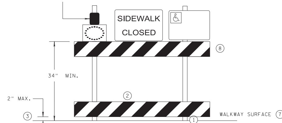
SIDEWALK BARRICADE
