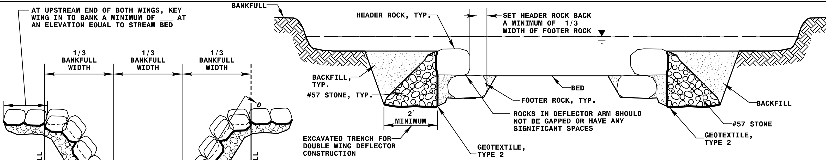
SECTION A-A
