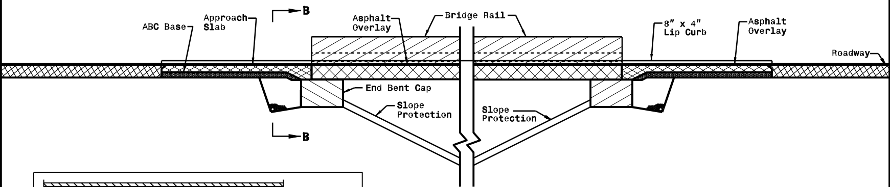
SECTION A-A
