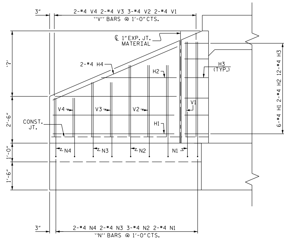
ELEVATION
